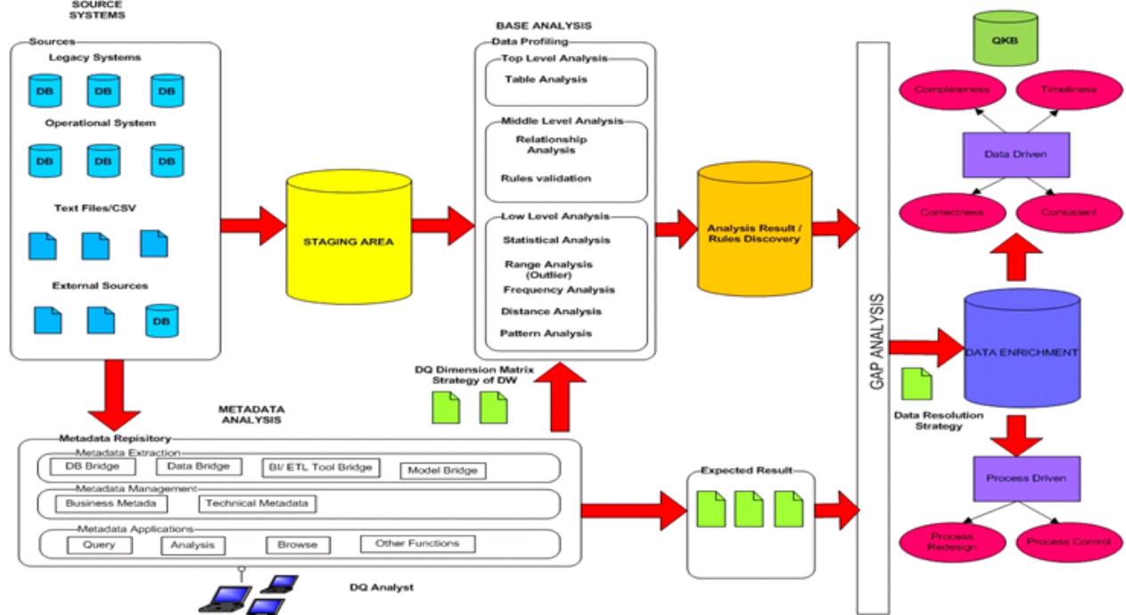
Fig. 1: DQ Framework
